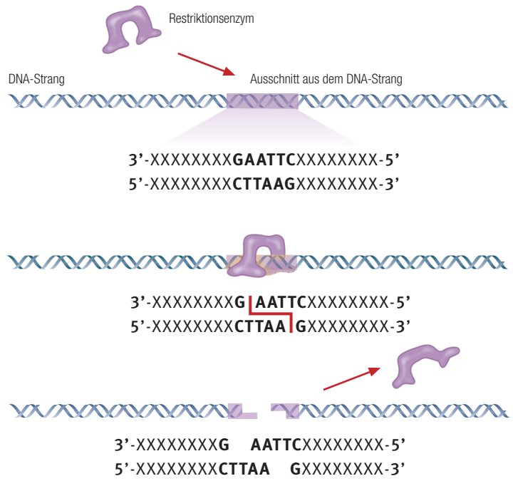
Grafik 2.1 Funktionsweise eines Restriktionsenzym
